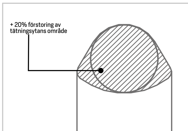
Fig 12 - Tätningringsprofil
