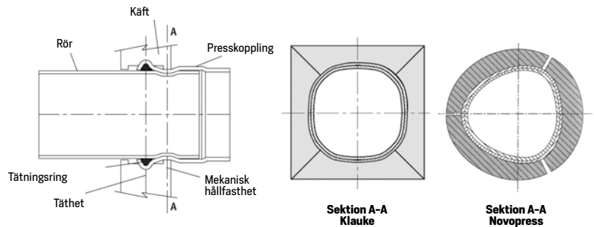
Fig 5 – Tvärsnitt genom en inoxPRES / steelPRES / aesPRES / marinePRES anslutning med kragen kvar i läge. Dimensionerna på 42–108 mm ger en definierad profil.
