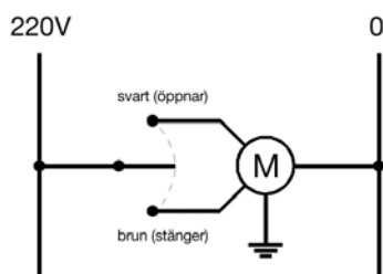
Kopplingsschema
