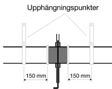
Exempel på horisontellt montage.
